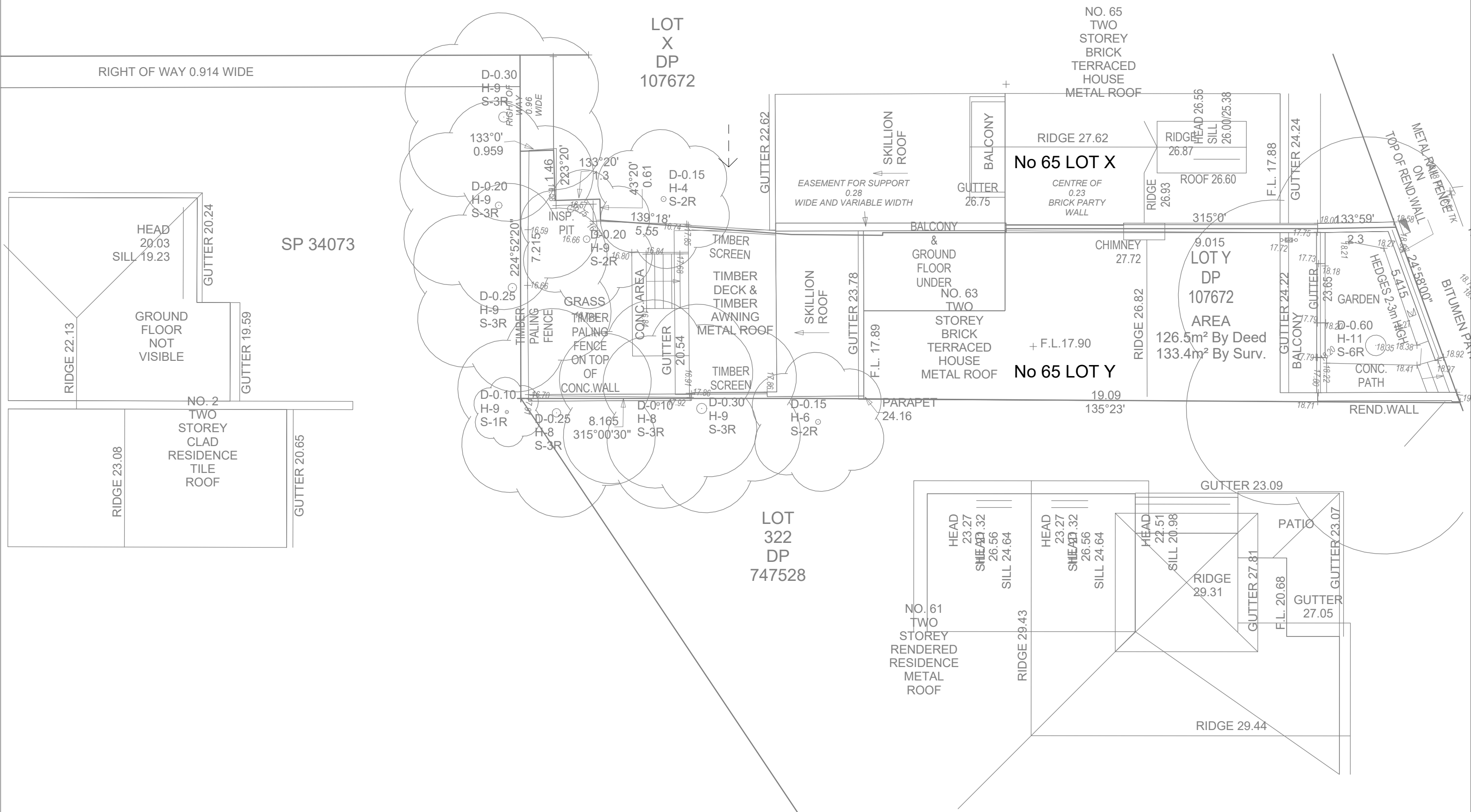
1 EXISTING SURVEY 1 : 100
